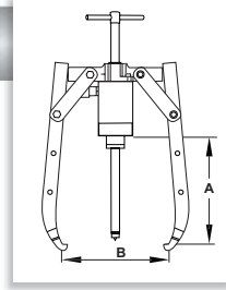
AP23xx 2/3 Leg Puller
